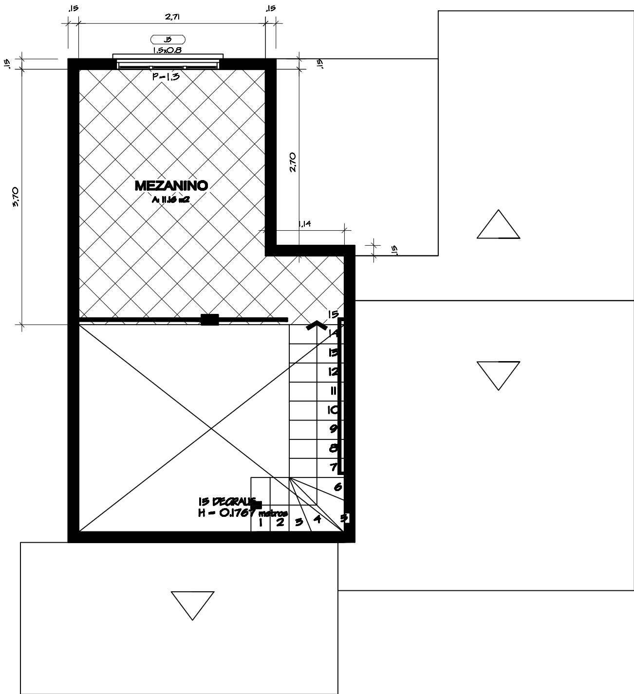
PLANTA BAIXA MEZANINO Escala 1 / 50
